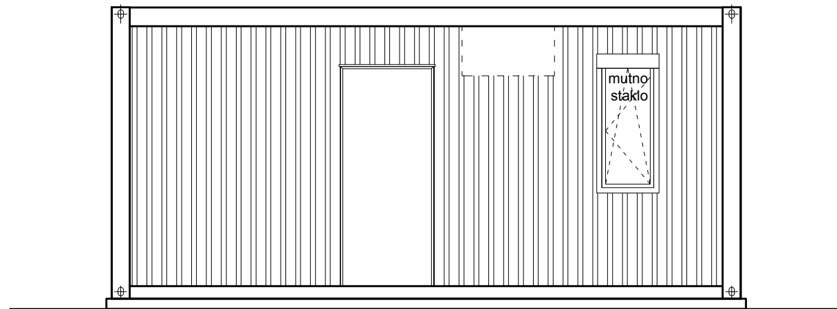
PROČELJE ISTOK
