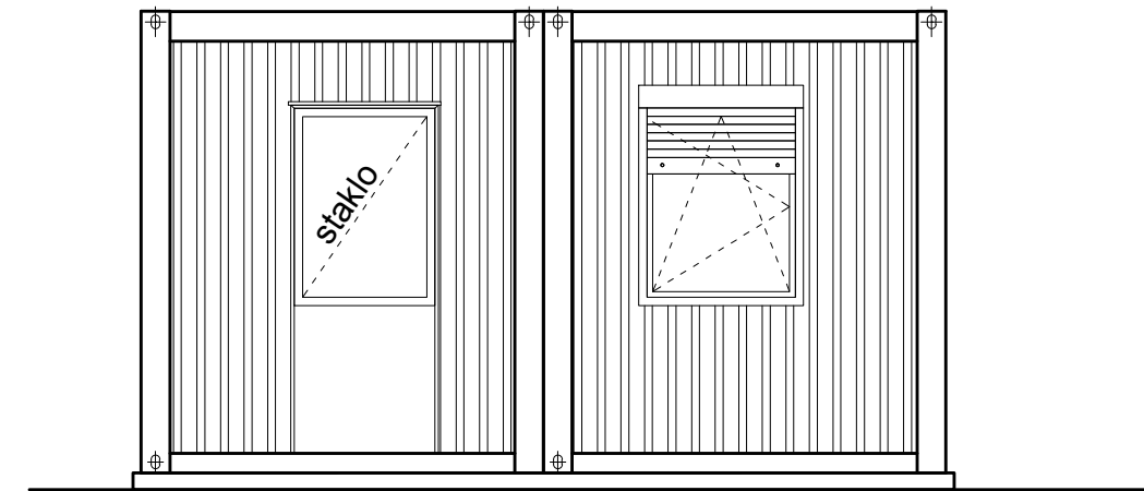
PROČELJE JUG
