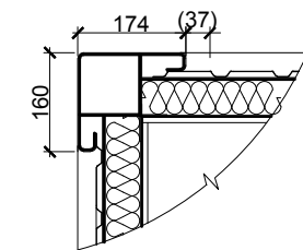
Detalj "A", 1:10
